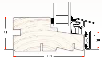
Álklæddur timburprófill
